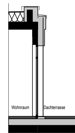
Schnitt Dachterrassenaustritt
